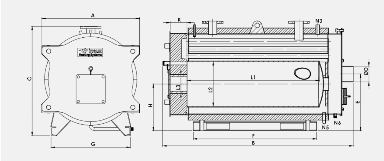
Внешний вид котла модели INSUZ PR 370 кВт – 847 кВт
